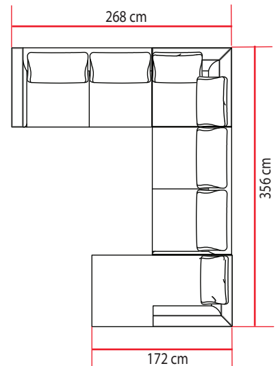
Modulacija SDUDL
